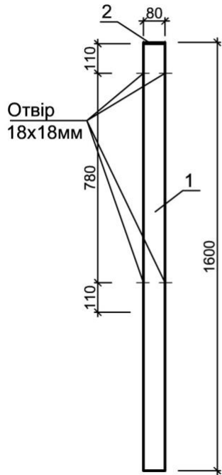
Стойка металева СТ-1
